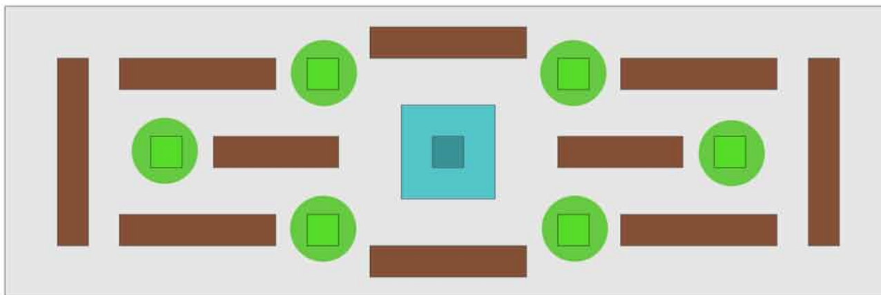
pianta | rapp. 1:100
